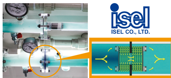
エレメント積層型ミキサー (MSE) 展示用機材と液体の流れを表したもの。
